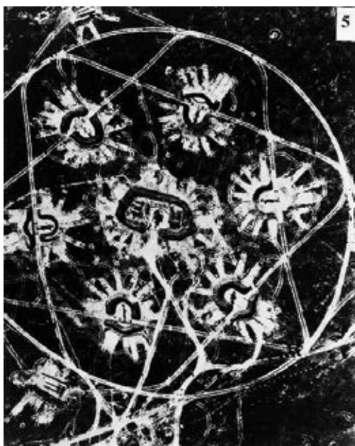
Διάταξη του συστήματος S-75 με τις θέσεις των εκτοξευτήρων πυραύλων περιμετρικά του radar ανίχνευσης κι ελέγχου πυρός SNR-75 ("Fan Song"). Λόγω του εξαγώνου σχήματος έφερε το προσωνύμιο «Άστρο του Δαυίδ». Πηγή: https://nsarchive2.gwu.edu/nsa/cuba_mis_cri/5.jpg (ανακτήθηκε στις 5-8-2022)
